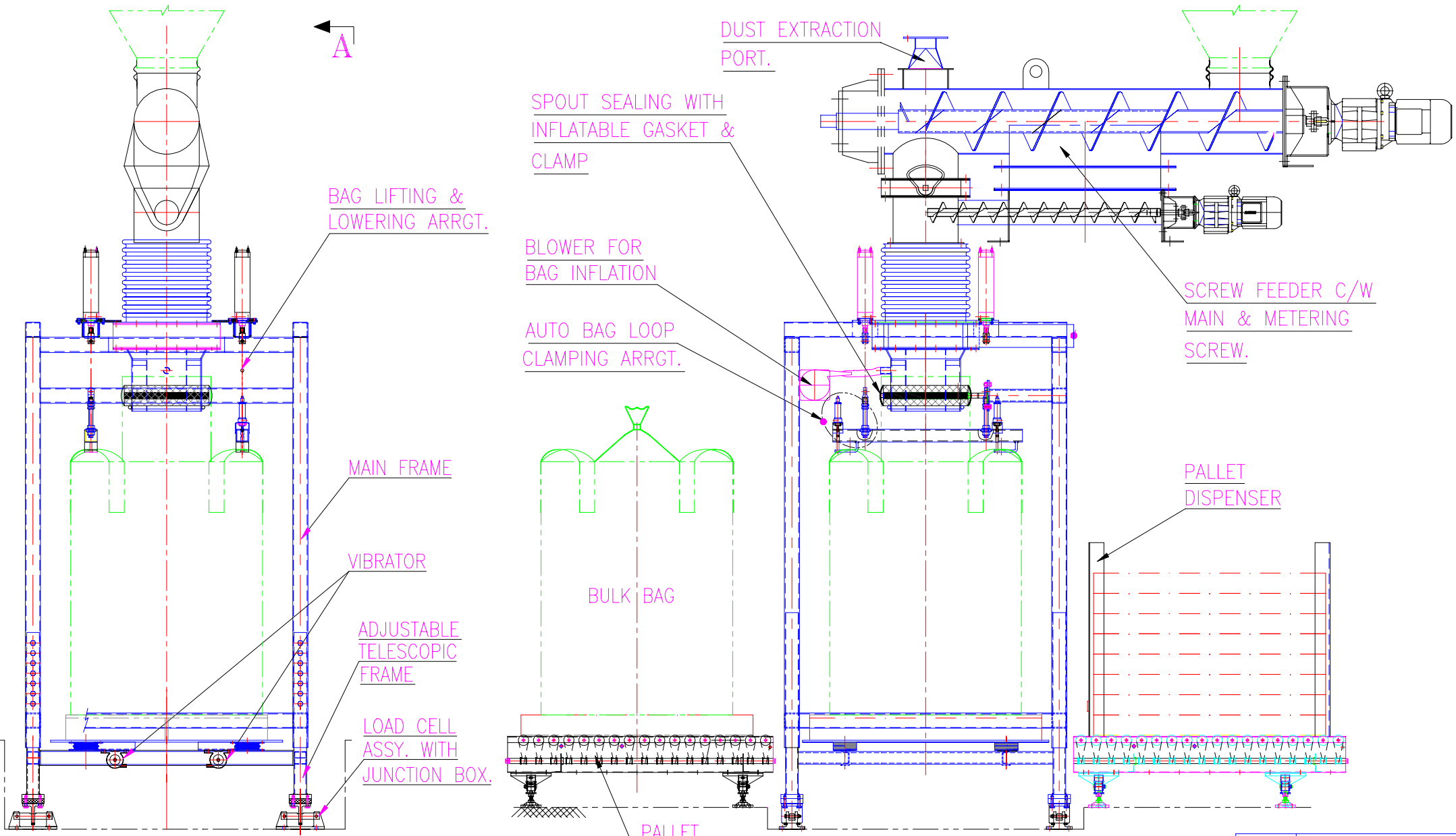
ELEVATION
